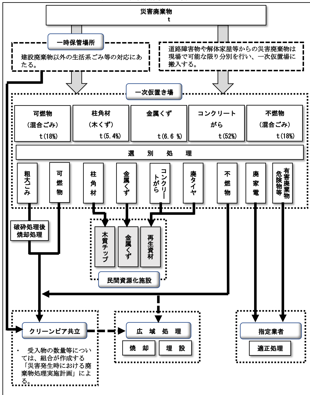
図 2-3 災害廃棄物の基本処理フロー
