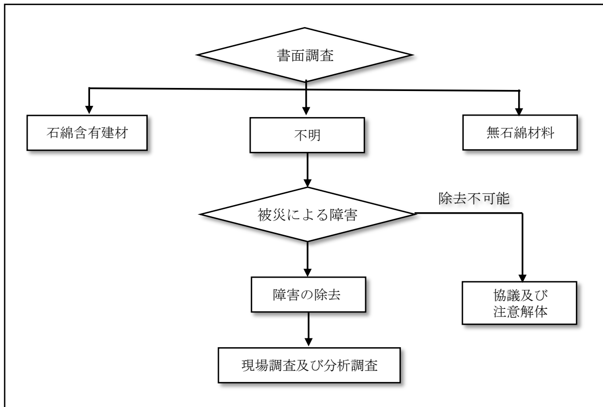
図 2-5 災害時における解体等事前調査
