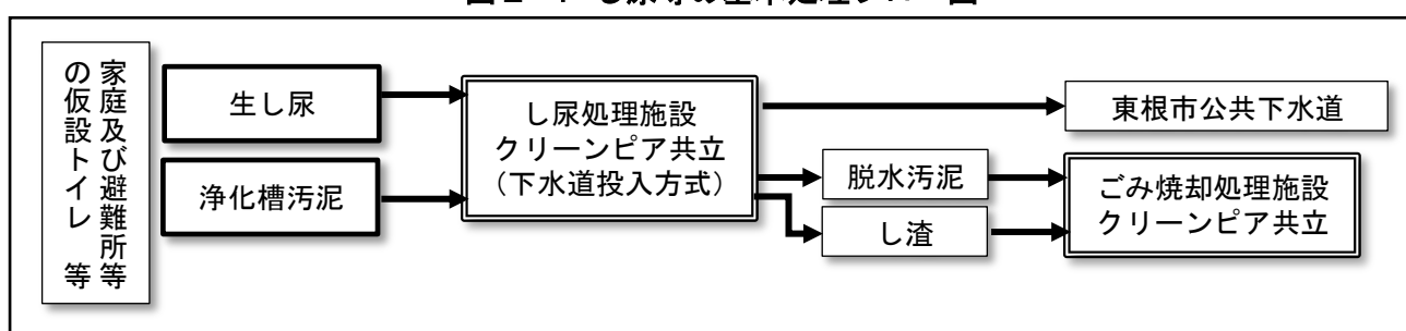
図2-1 し尿等の基本処理フロー図
